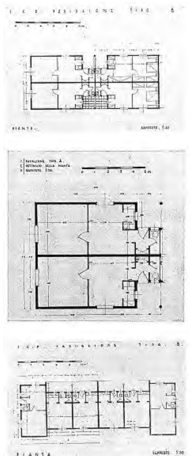
Piante di alloggi, da «L'Ingegnere», 1936, n. 9
